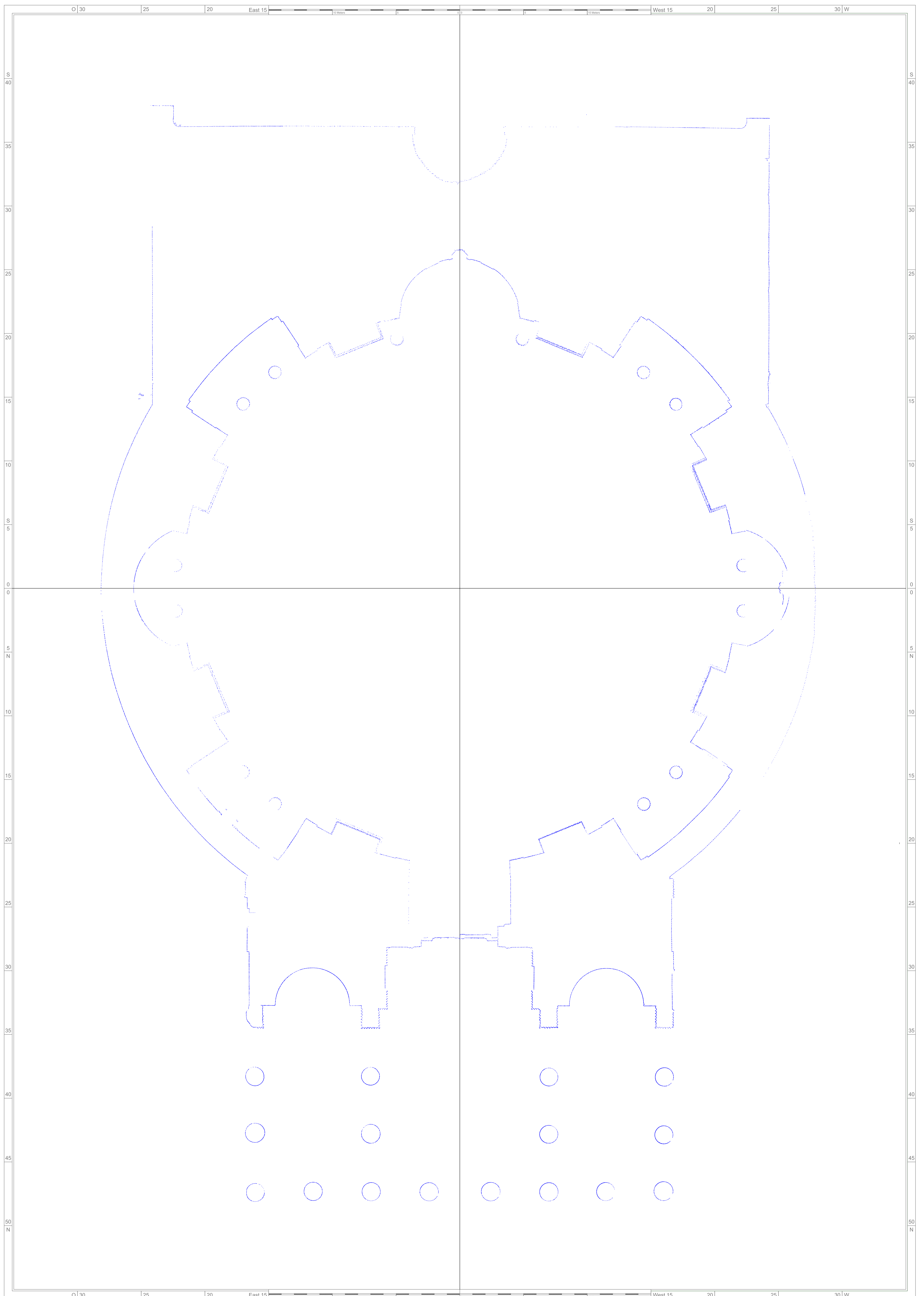
Section 07 (7 meter above z=0, slice thickness 0,10 m)
